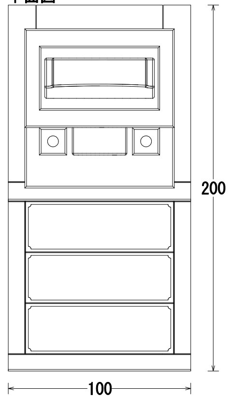
平面図
