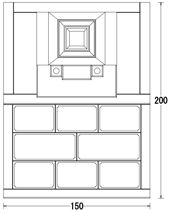
平面図
